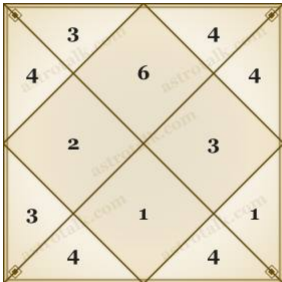
Mars
