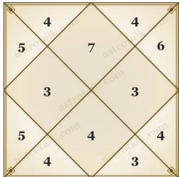
Venus
