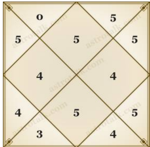
Moon
